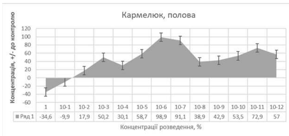
Рис. 9 Біологічна активність лектинів половки пшениці озимої сорту Кармелюк в системі біотесту залежно від концентрації
