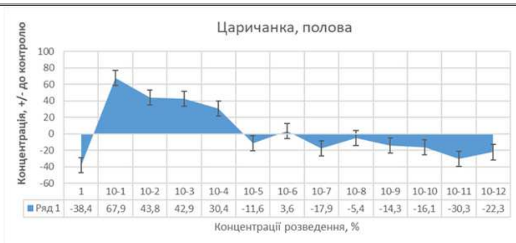
Рис. 8 Біологічна активність лектинів половки пшениці озимої сорту Царичанка в системі біотесту залежно від концентрації
