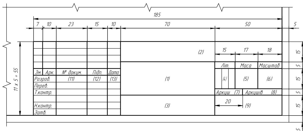
Рисунок 1 – Основний напис на аркушах креслеників
