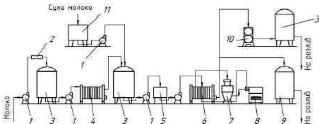
Рис.1 Машинно-апаратна схема виробництва пастеризованого молока
