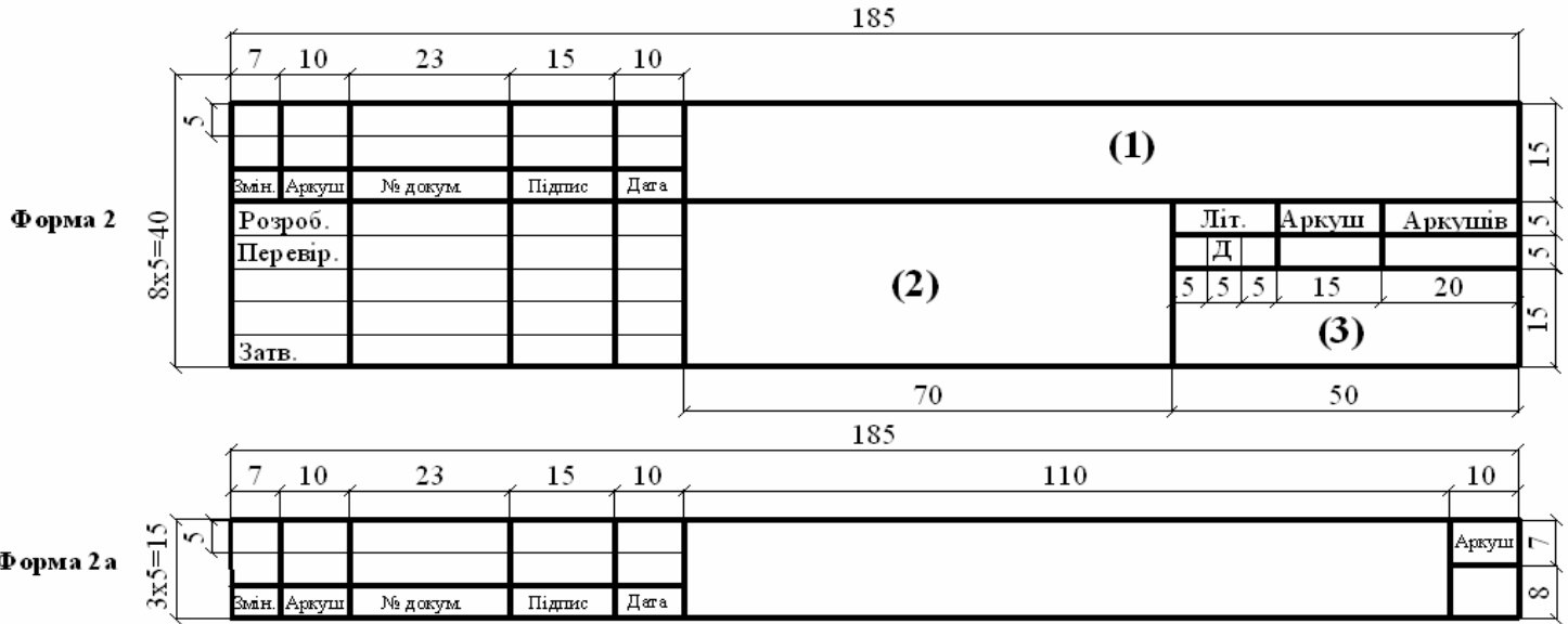
Рис. Е.1. Форма основного напису: Ф2 - на аркуші «Зміст» пояснювальної записки, Ф2а - наступних аркушах записки:
