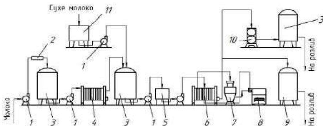
Рис.1 Машино-апаратна схема виробництва пастеризованого молока
