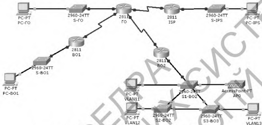
Рис. 1. Варіант топології комп'ютерної мережі.
