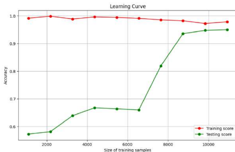
Рис 4. Крива навчання для ансамблевого метода
