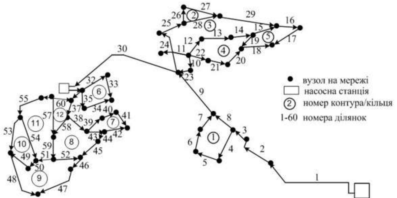
Рис. 1. Схема мережі транспортування води
