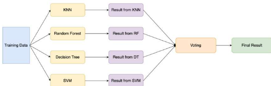
Рис. 2. Ансамблевий метод голосування
