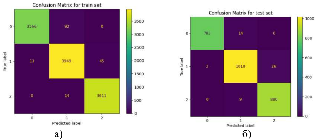
Рис 3. Матриця помилок для: а) тренувального набору для ансамблю; б) тестового набору для ансамблю
