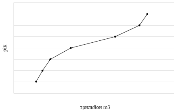
Рис. 1. Глобальне використання прісної води [2]
