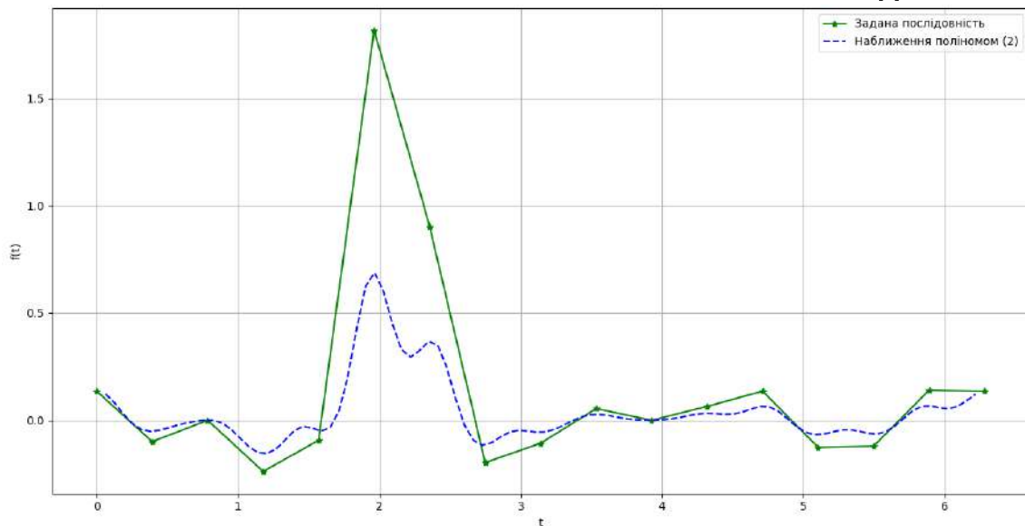
Рис. 2. Візуалізація наближення тієї ж функції поліномом (2), тільки з більшою кількістю відліків
