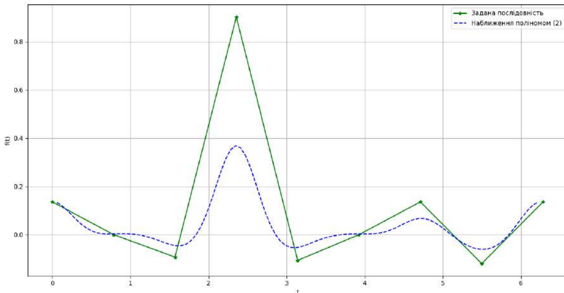
Рис. 1. Візуалізація наближення функції поліномом (2)
