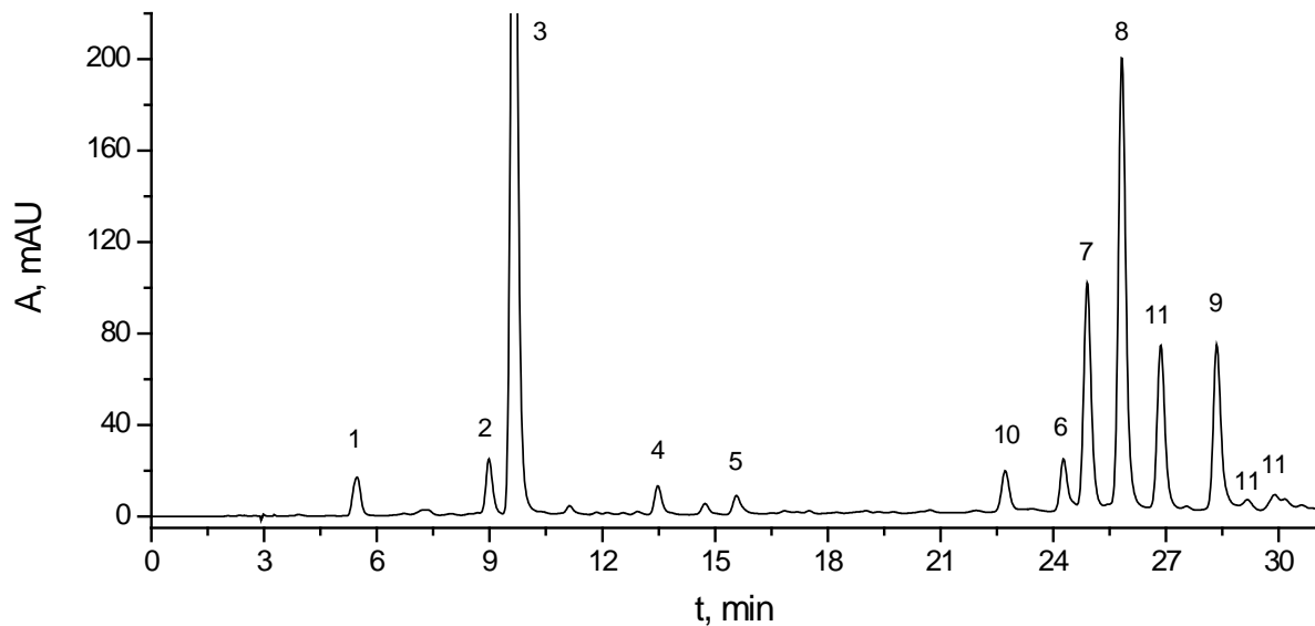
Рис. 1. Хроматограмма экстракта листьев топинамбура. Колонка Hyperpack Basic ODS, 5 мкм, 4.6x150 мм; линейный градиент 7-23% ацетонитрила в 0,05% растворе уксусной кислоты за 30 мин при скорости 0,75 мл/мин; детекция при 325 нм:
