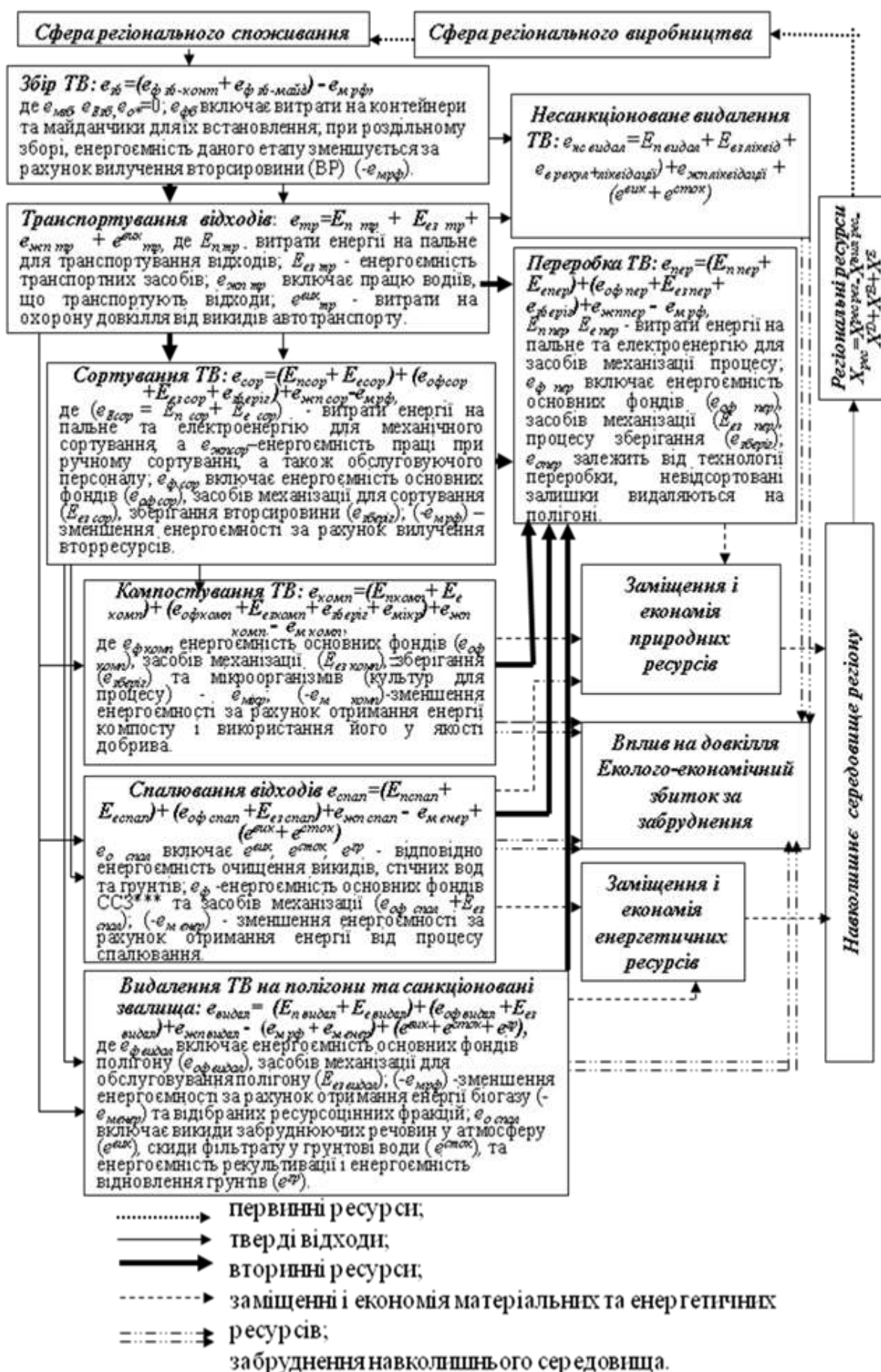
Рис.1 – Балансова схема життєвого циклу твердих відходів регіону
