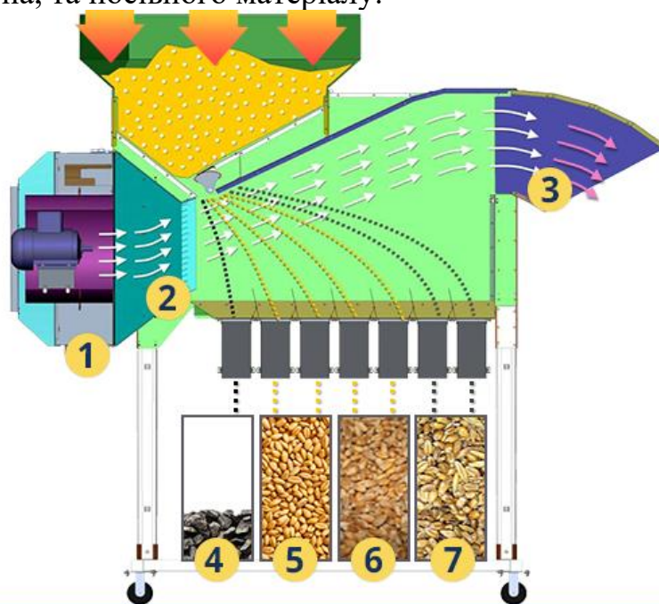
Рисунок 4. – Аеродинамічний сепаратор зерна до 2т.
