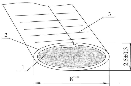
1-шихтовий наповнювач; 2-сталева оболонка; 3- рифлення
