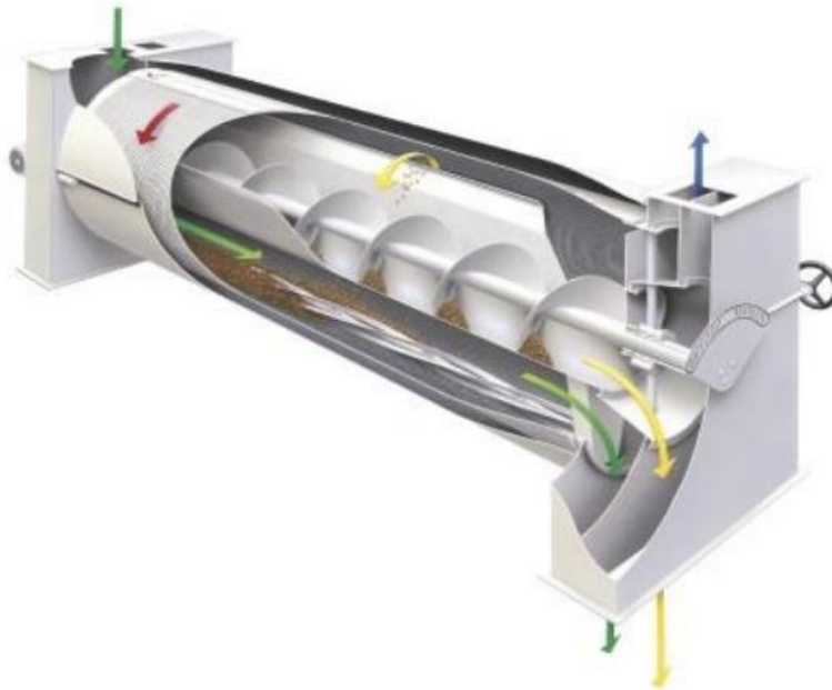
Рисунок 3. – Барабанний трієр для очищення зерна
