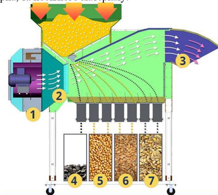
Рисунок 4. – Аеродинамічний сепаратор зерна до 2т.
