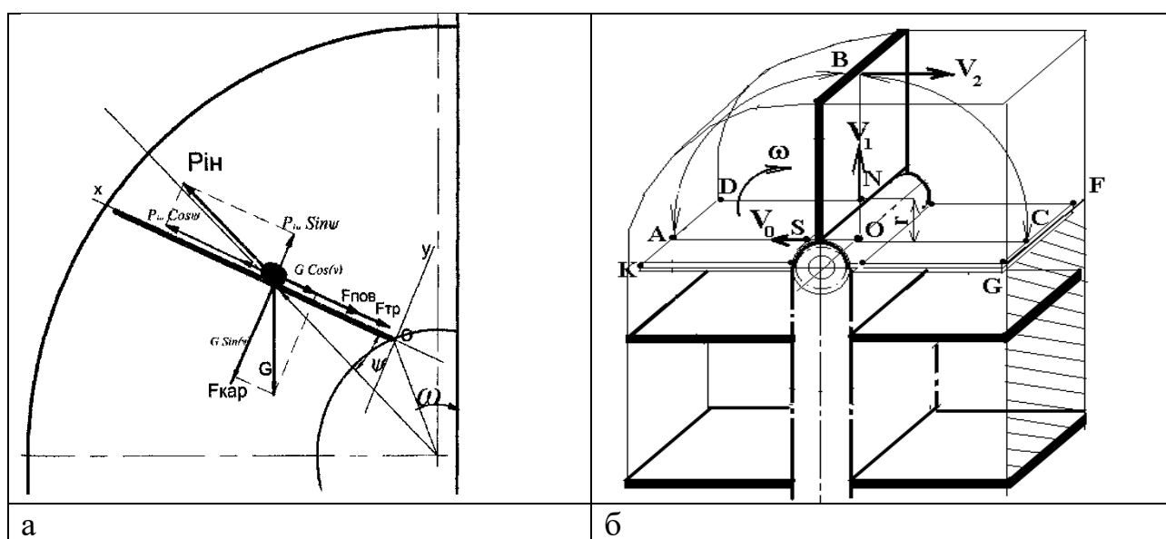
На зернину діють сили: G = mg – вага зерна; N – нормальна реакція
