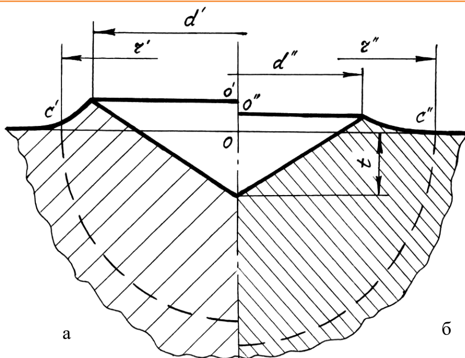
Рисунок 1. – Розповсюдження деформації і профіль відбитка при втисненні конічного індентора в метал з низькою (а) і високою (б) пластичністю.
