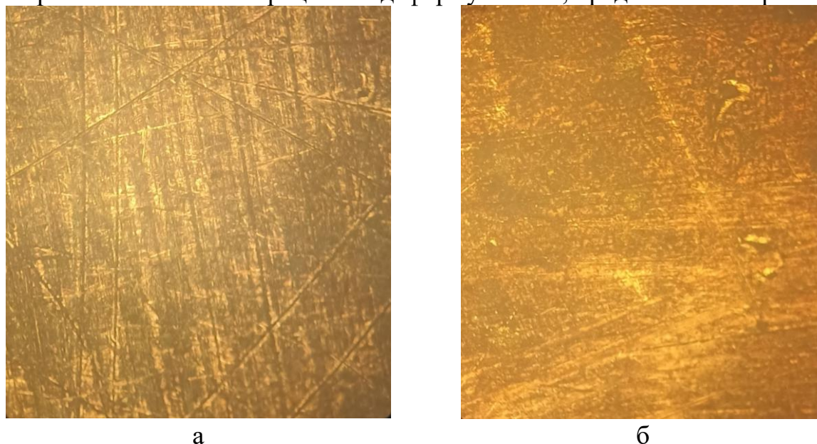
Рисунок 2. – Фотографія мікроструктури зразків поверхні бронзи CuSn5Zn5Pb5 за умови збільшення \times 100 : а – без деформування; б – вібраційне деформування
