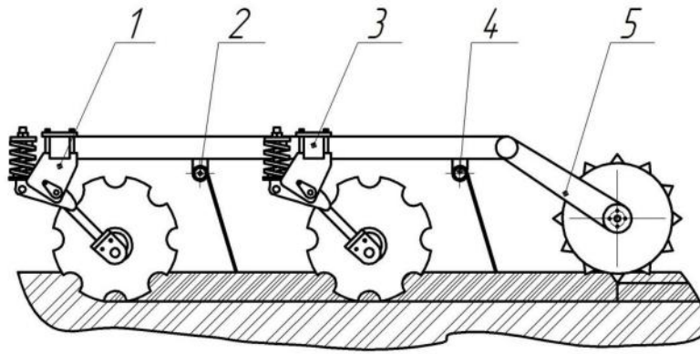
Рисунок 3. – Дискова борона Рубін 9 600/KU фірми Lemken (ФРН)
