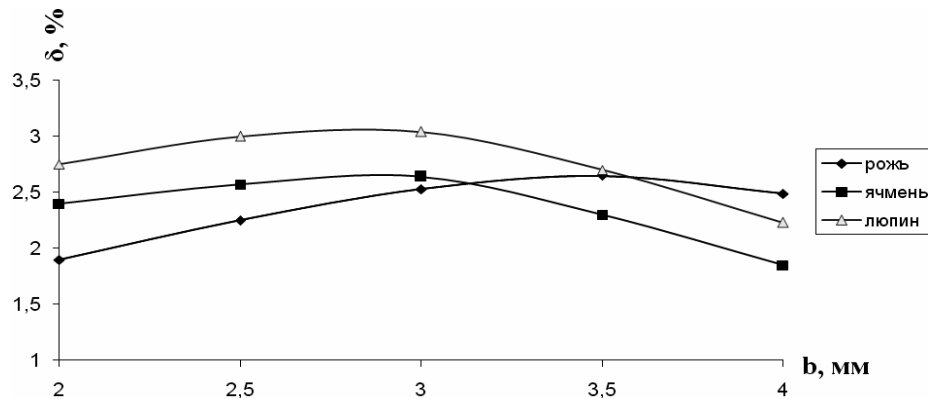
Рисунок 1. – Зависимость неравномерности распределения материала по семяпроводам от высоты сферического отражателя
