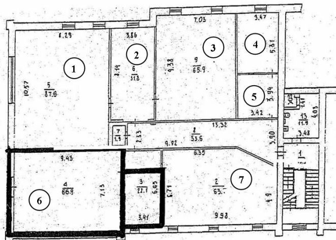
Рисунок 1.1 – План поверху офісної будівлі за варіантом № 1
