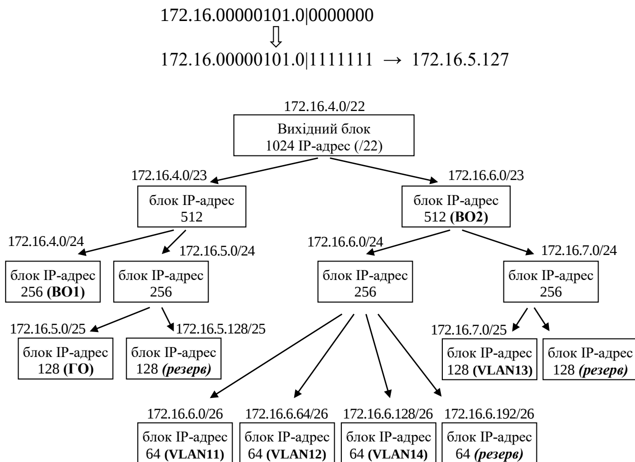
Рисунок 2.3 – Схема IP-адресації проектованої комп'ютерної мережі
