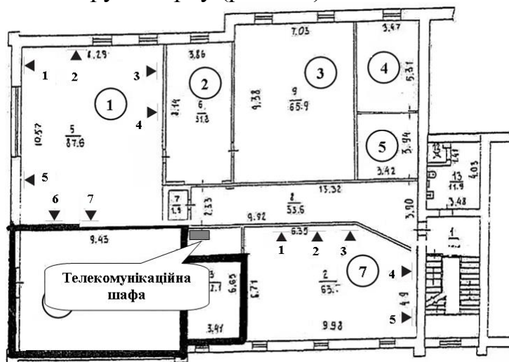
Рисунок 1.3 – Варіант розміщення телекомунікаційної шафи
