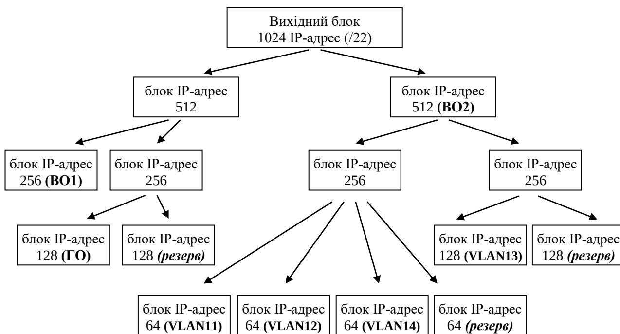
Рисунок 2.1 – Схема розподілу вихідного блоку IP-адрес
