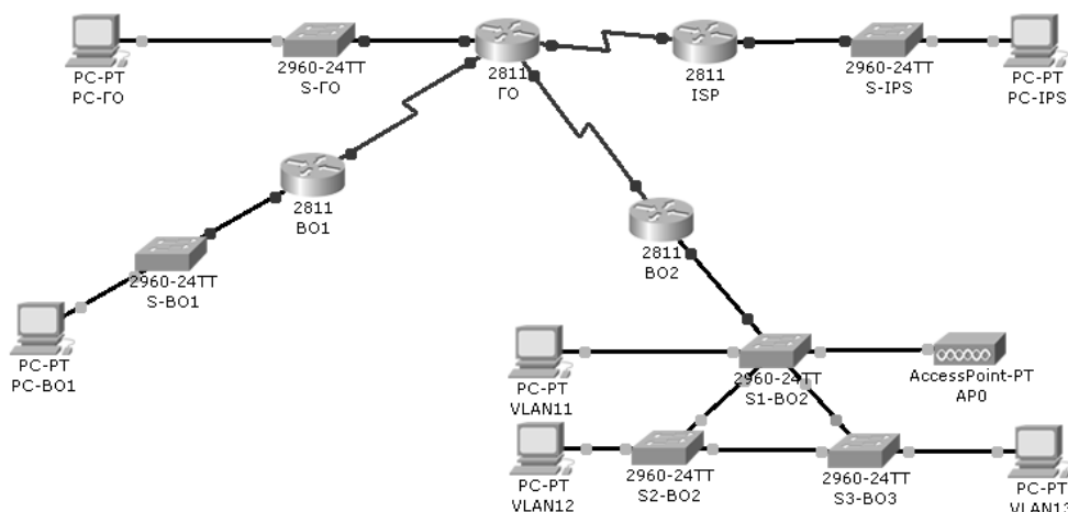
Рисунок 1 – Варіант топології комп'ютерної мережі
