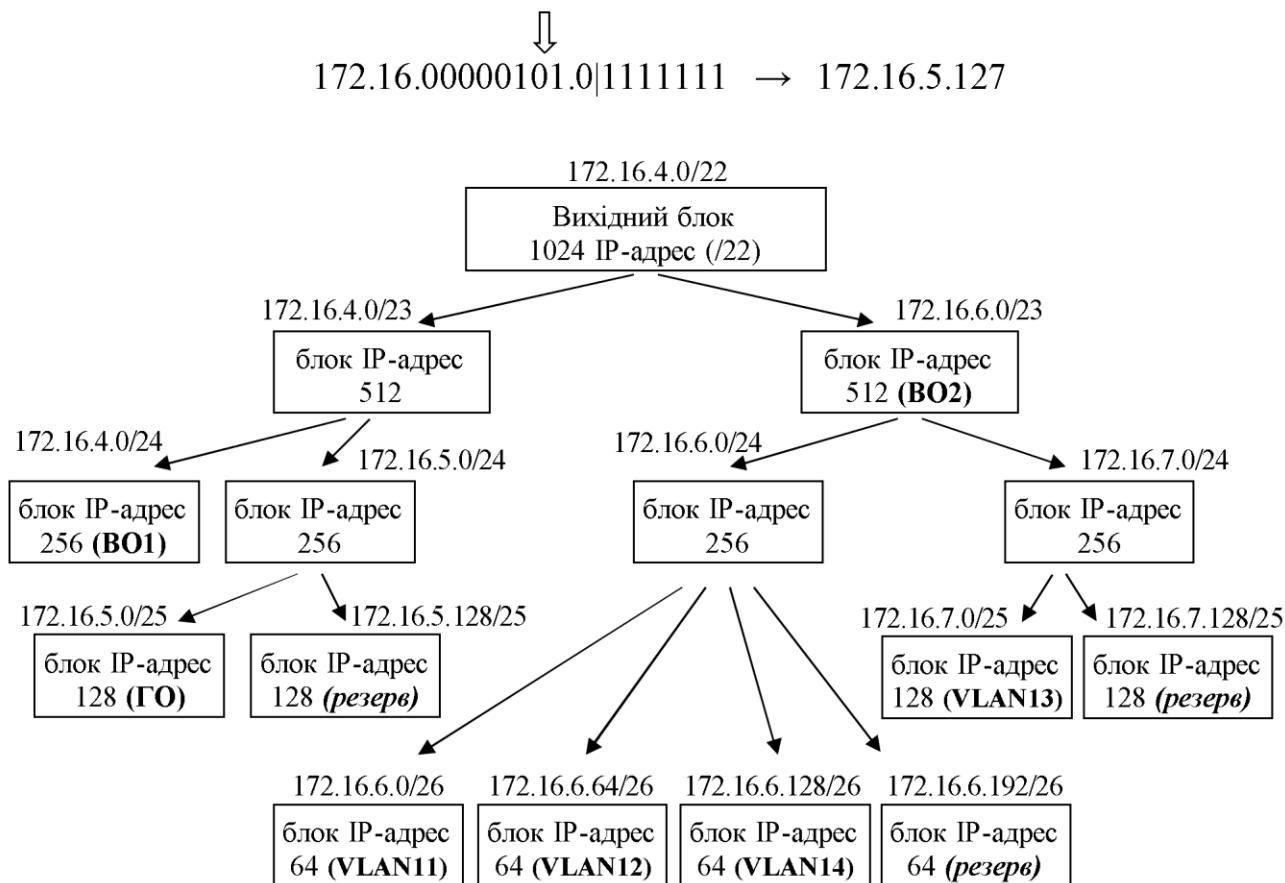
Рисунок 2.3 – Схема IP-адресації проектованої комп'ютерної мережі
