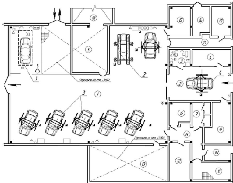
Рисунок 6. – приклад зони ТО, ремонту та передпродажної підготовки автомоболів [1]: 1–ділянка ТО, ПР та передпродажної підготовки автомобілів, 2 – ділянка приймання-видачі автомобілів, 3 – шиномонтажна ділянка, 4 – приміщення майстра-приймача (приміщення для оформлення документів), 5 – склад запасних частин, 6 – каса, 7 – санітарні вузли, 8 – коридор, 9 – диспетчерська, 11 – сходова клітка, 12 – буфет, 13 – приміщення для відпочинку клієнтів СТО, 14 – коридор, 15 – склад гарантійного запасу, 16 – суміжне приміщення, 17 – склад зареklamованих запасних частин, 18 – складське приміщення. Експлікація постів: 1 – спеціалізований пост перевірки та регулювання системи освітлення та світлової сигналізації автомобілів, 2 – спеціалізований пост для перевірки та регулювання кутів установлення коліс автомобілів, 3 – універсальні пости ТО, ПР та передпродажної підготовки автомобілів, 4 – пост приймання автомобілів.
