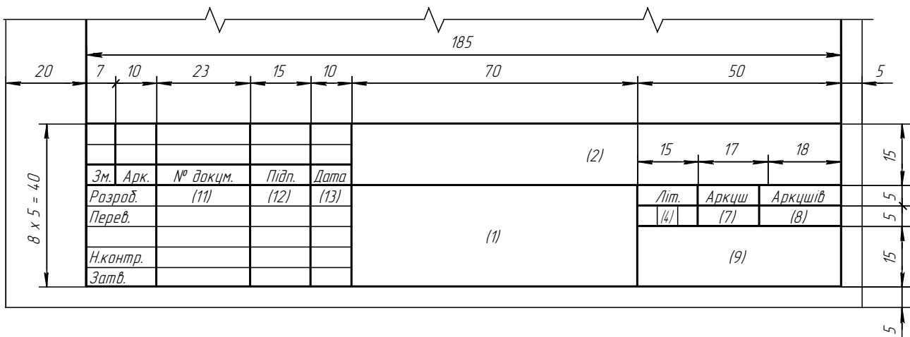
Рисунок 4 – Основний напис першого аркуша текстового документу (форма 2)
