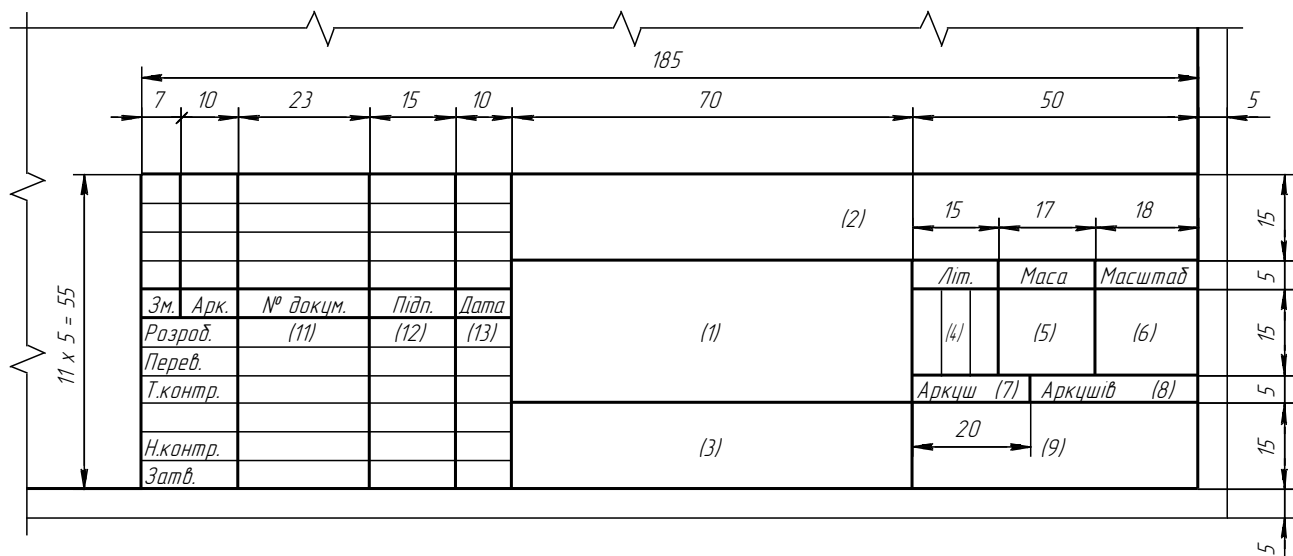
Рисуюнок 3 – Основний напис на аркушах креслень
