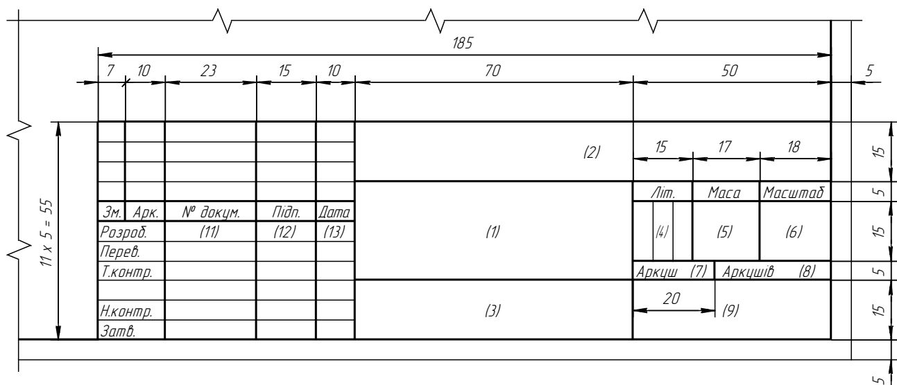
Рисунок 3 – Основний напис на аркушах креслень (форма 1)
