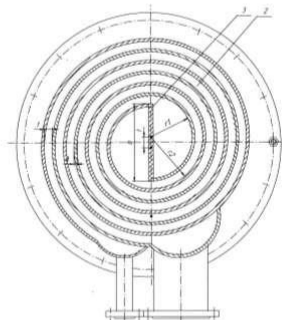
Рисунок 8 – Спіральний теплообмінник:
