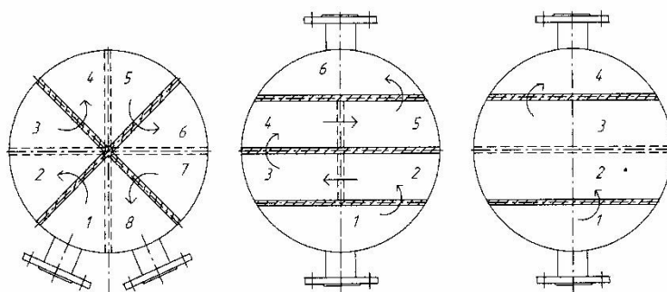
Рисунок 5 – Варіанти розміщення перегородок у кришці багатоходових теплообмінників
