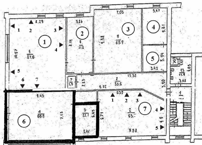
Рисунок 1.2 – План поверху офісної будівлі з зазначенням місць розміщення мережевих розеток
