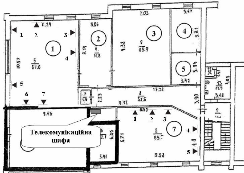
Рисунок 1.3 – Варіант розміщення телекомунікаційної шафи
