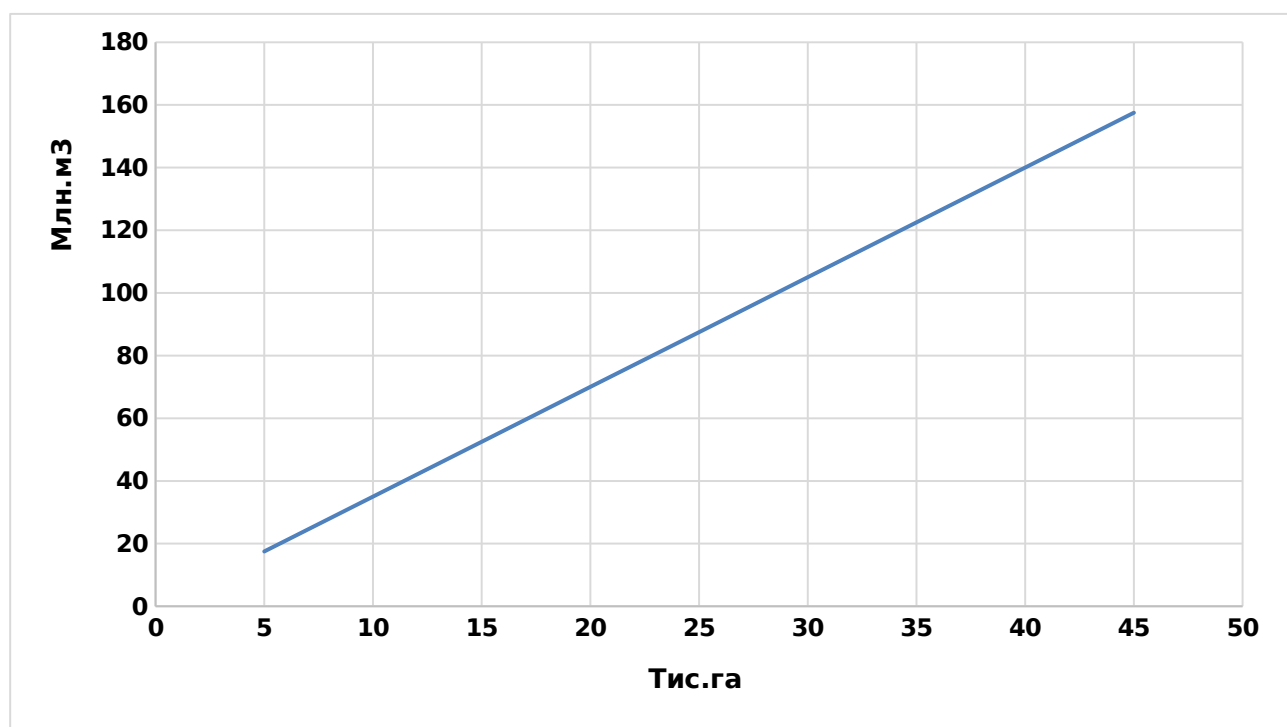
Рис. 1.2 - Лінійна залежність обсягів середнього багаторічного додаткового випаровування від площі водного дзеркала для Дніпропетровської області
