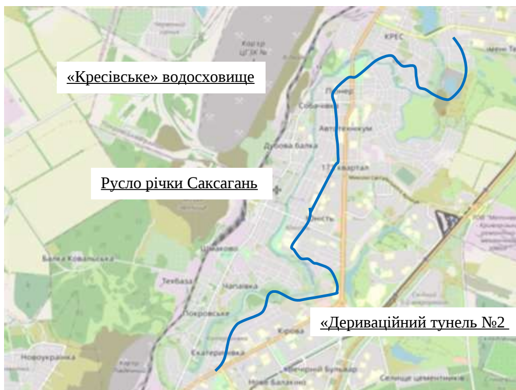
Рисунок 1.1 – Ділянка русла річки Саксагань від «Кресівського»
